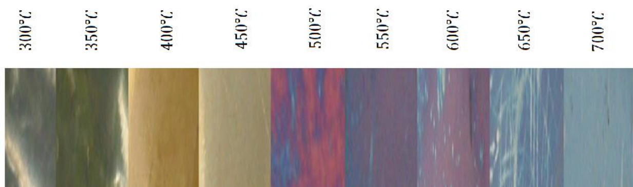
Рис. 3.2. Шкала залежності кольору від температури
