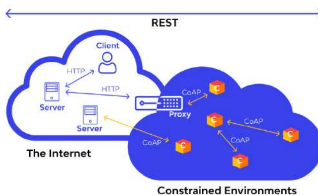
Рисунок 3.9 – Архітектура CoAP
