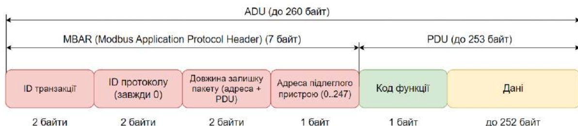
Рисунок 4.8 – Структура пакету протоколу Modbus TCP
