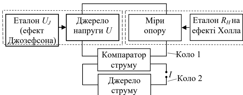
Рис. 4.16. Установа для відтворення «квантового» ампера
