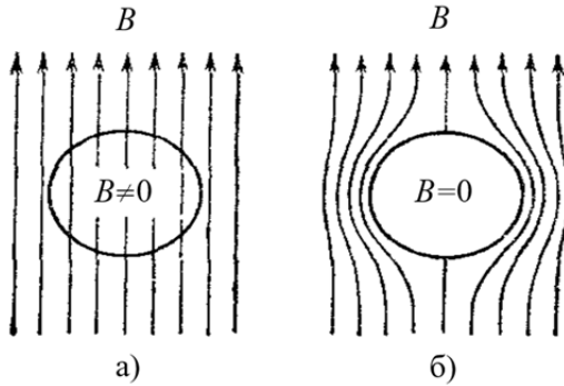
Рисунок 2.4. Ілюстрація ефекту Мейснера
