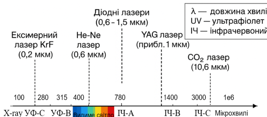
Рисунок 3 – Спектр електромагнітного випромінювання лазерів
