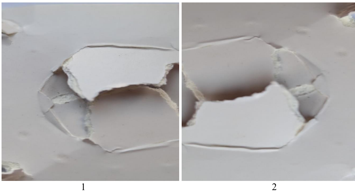
Рисунок 11 – Зразки лакованого картону після досліджень на продавлювання: 1 – SinarVanda GC1 – 245 г/м 2 ; 2 – SinarVanda GC1 – 280 г/м 2
